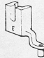
オサエアシ E Presser Foot E (φ1.6) 154089-001
