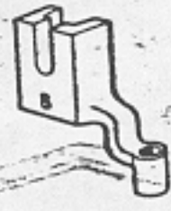
オサエアシ B Presser Foot B (φ4) 152636-001
